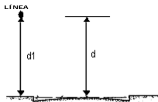
Figura 6. Distancias "d" y "d1" en cruces y recorridos de vías
