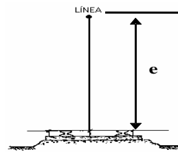
Figura 7. Distancia "e" en cruces con ferrocarriles sin electrificar
