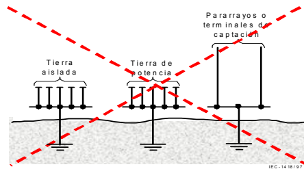
Figura 12. Puestas a tierra separadas o independientes
